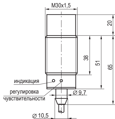
Габаритный чертеж
